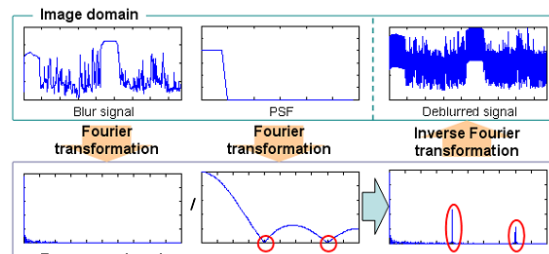
図 3 1次元信号でのぶれ信号復元
