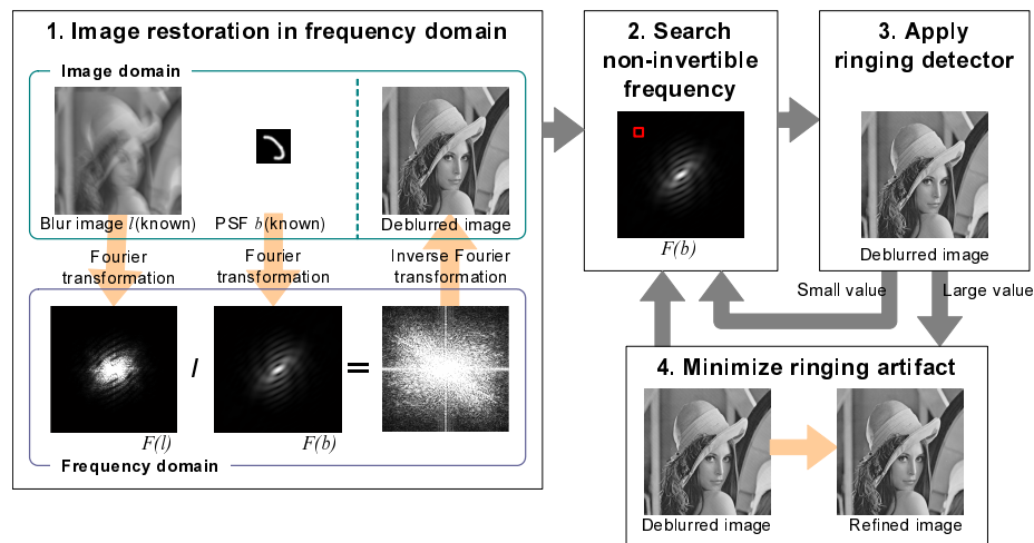
図6 リンギング検出器を用いたぶれ画像復元の流れ
