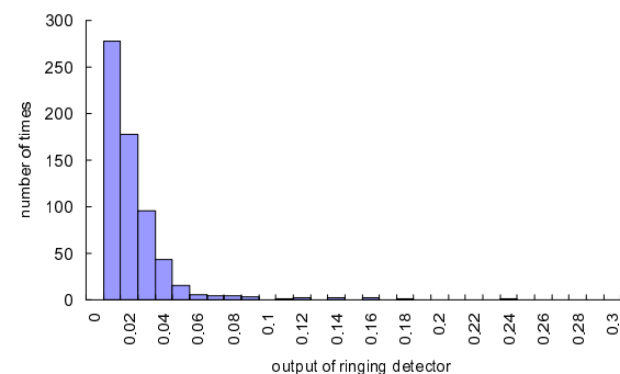
図7 リンギング検出器の出力のヒストグラム ( a=0.125, b=0.125 )
